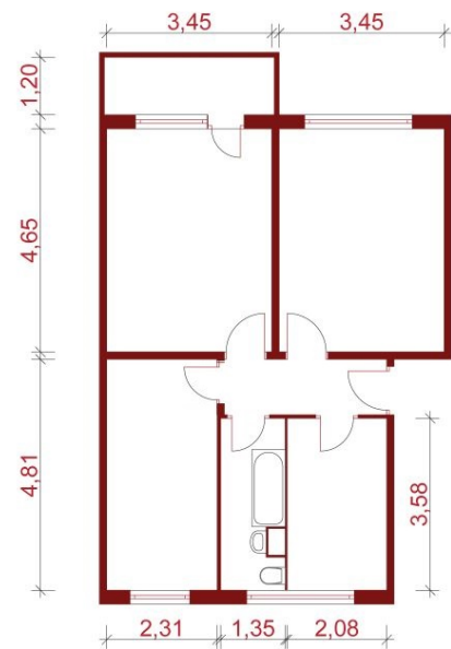
Grundriss
